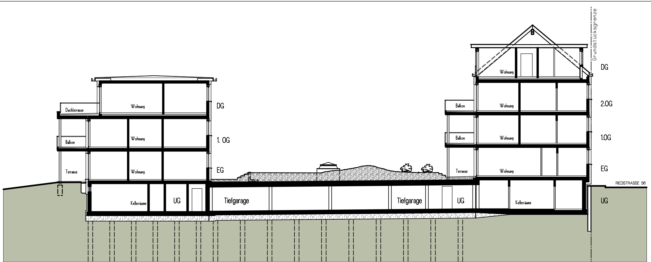
SCHNITT B - B HAUS B
